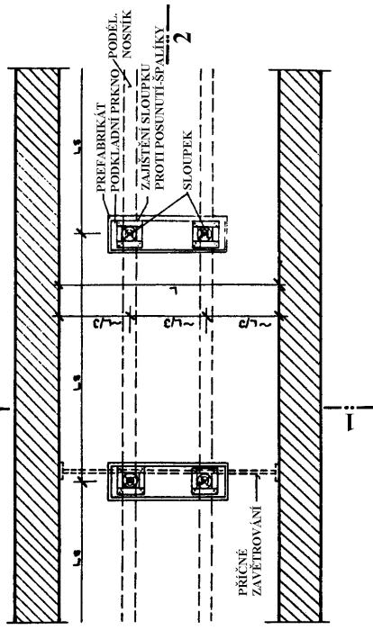
PŮDORYS
